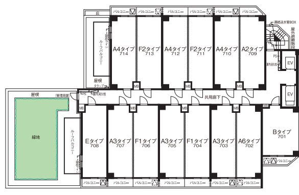
7階平面図
