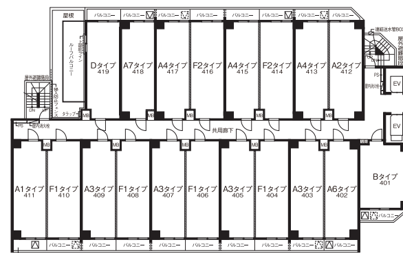
4階平面図
