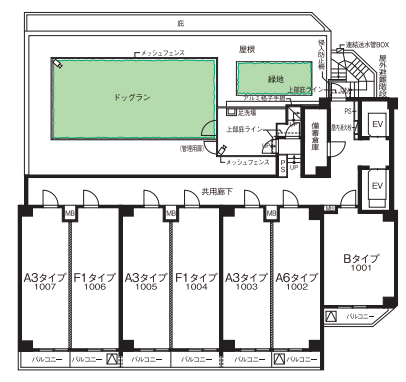
10階平面図
