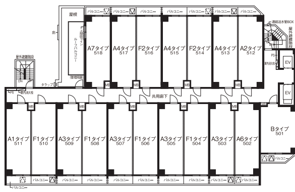
5階平面図
