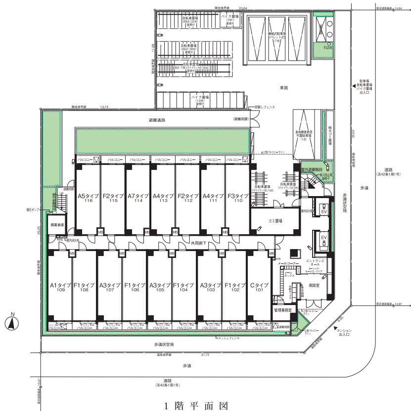
1階平面図
