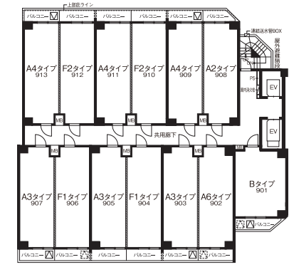
9階平面図
