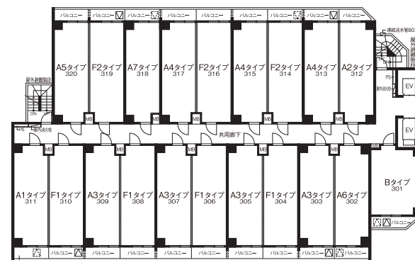
3階平面図
