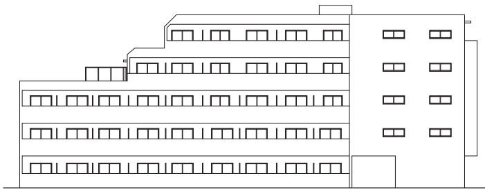
西立面图
