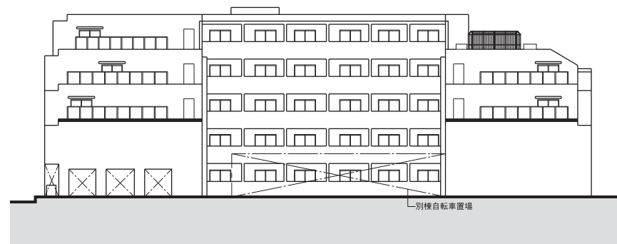
東立面图
