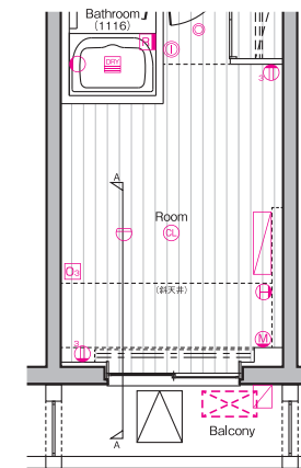
426号室 部分図
