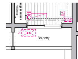
501号室 部分図
