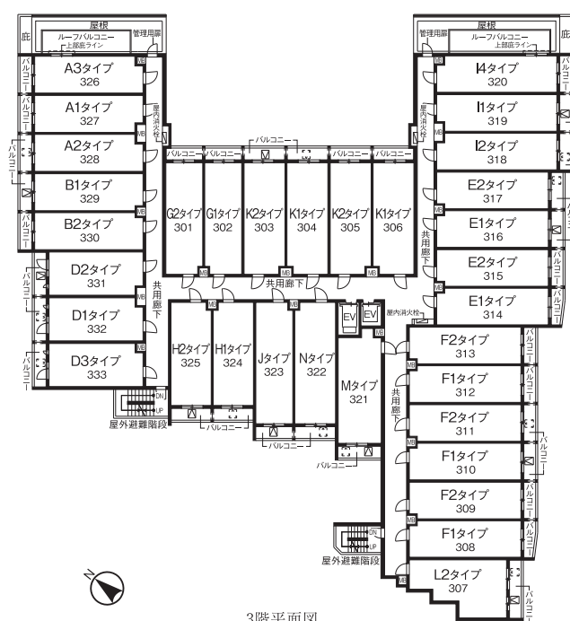
3階平面図
