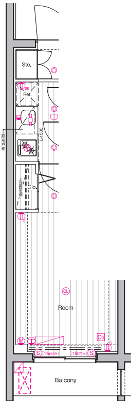
125・227号室 部分図
