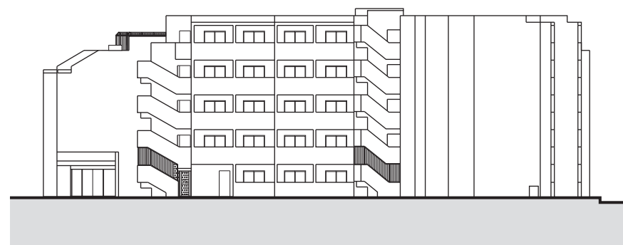
西立面图
