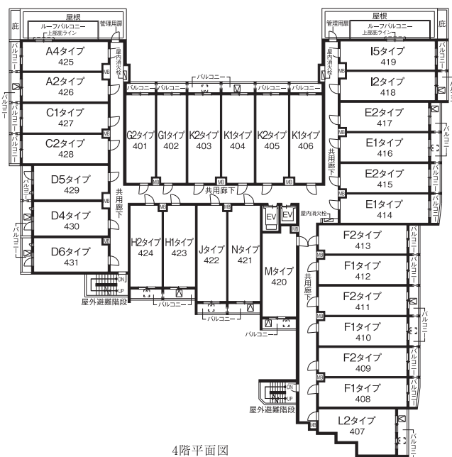
4階平面図
