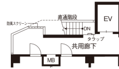
5階 階段部分図
