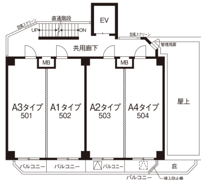
3階平面図
