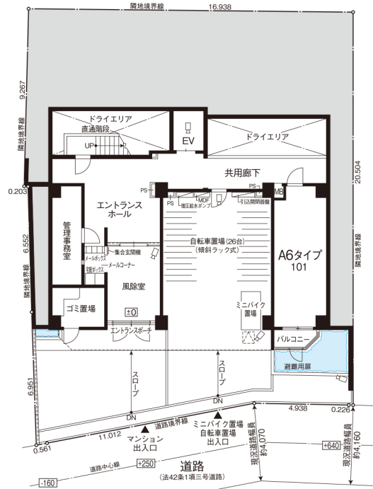
B2階平面図
