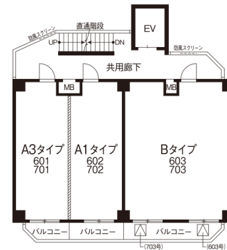
4階・5階平面図
