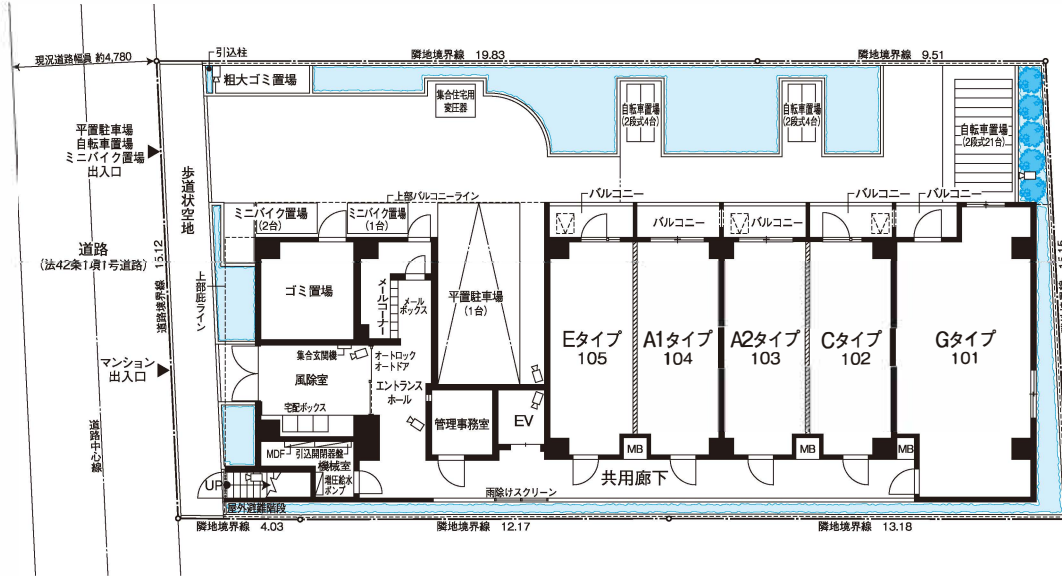
[1F平面図・敷地配置図] SCALE:約1/250
