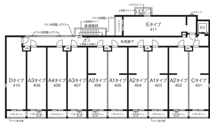
4階平面図
