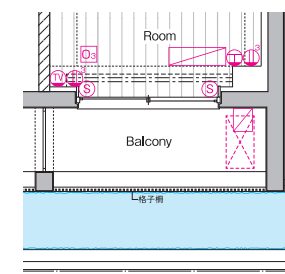
■101号室部分図
