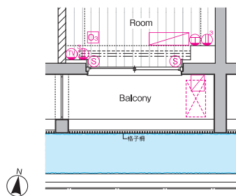
■103・105号室部分図
