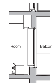
■A-A 断面図
