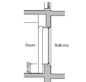
■A-A 断面図
