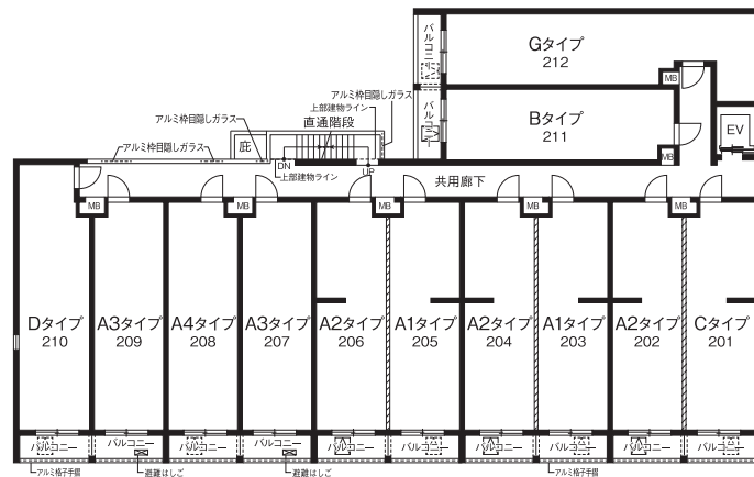
2階平面図
