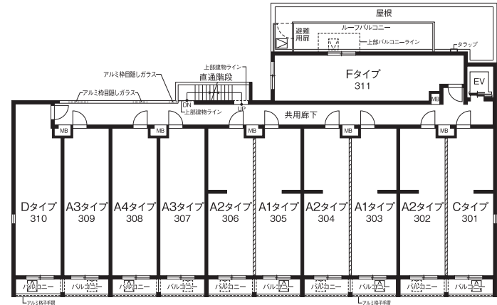
3階平面図
