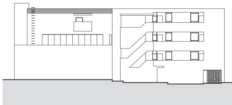
北立面图
