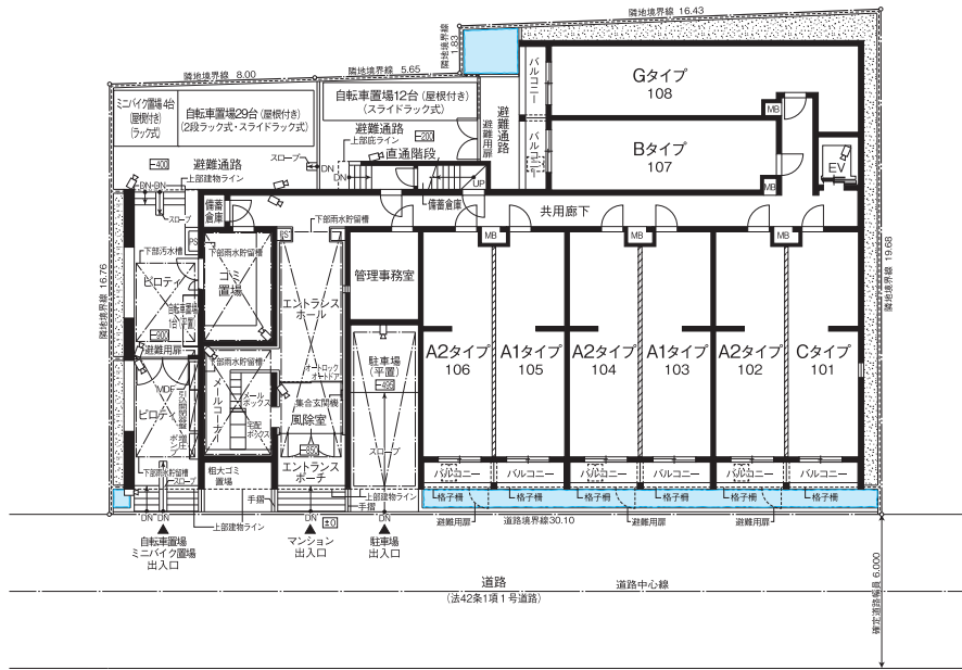
防犯カメラ 1階平面図
