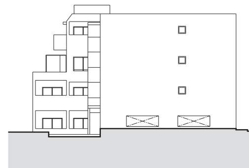
西立面图
