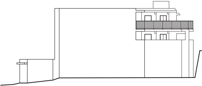
东侧立面图
