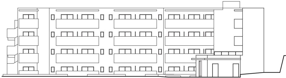
南侧立面图
