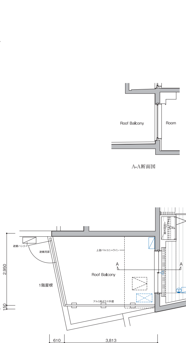
201号室部分図
