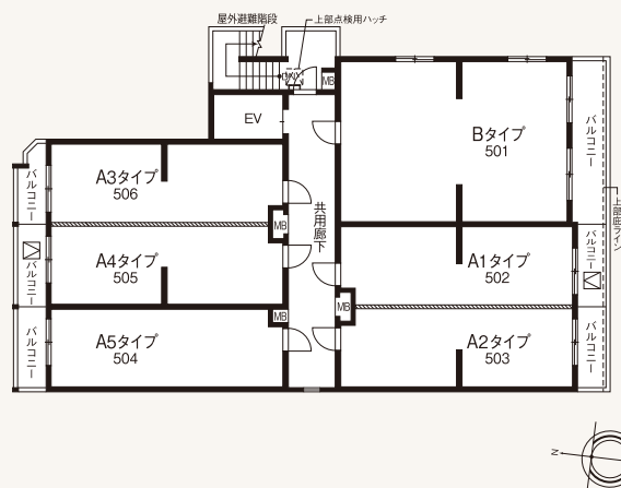
5階平面図
