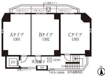
13階平面図
