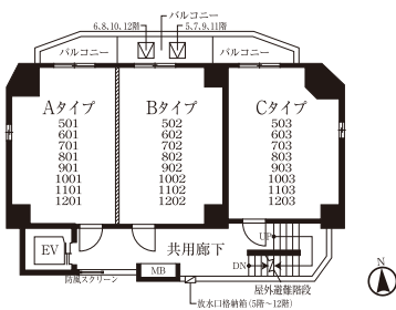
5-12階平面図
