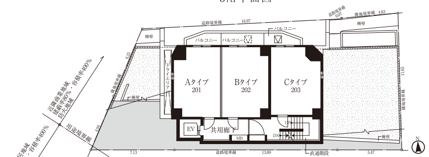
2階平面図
