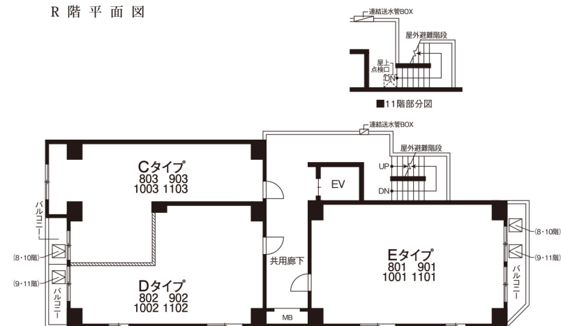
8 ~ 1 1 階 平 面 図
