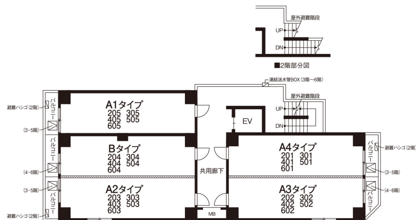
2 ~ 6 階 平 面 図
