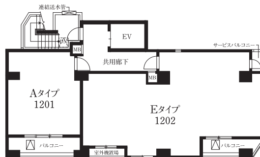
12階平面図
