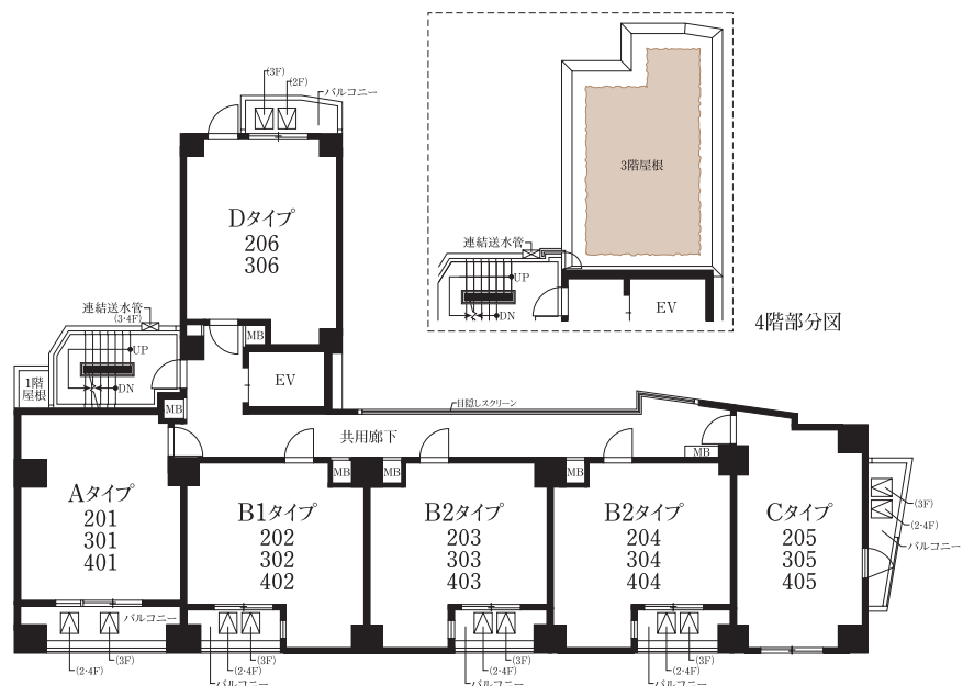
2～4階平面図
