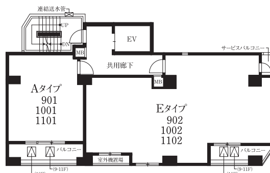
9～11階平面図
