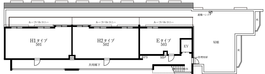
5階平面図
