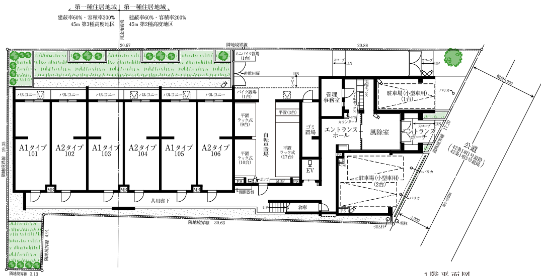
1階平面図
