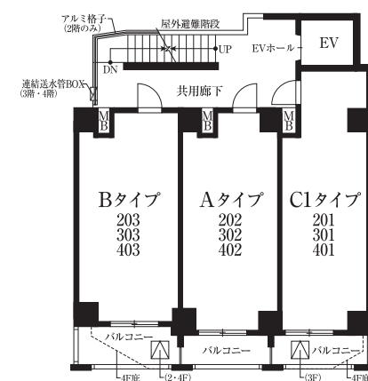
2~4階平面図
