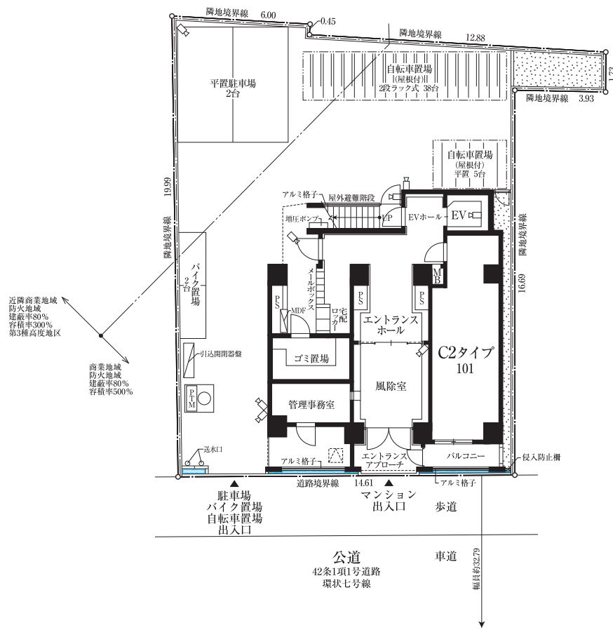
配置図/1階平面図 □ 防犯カメラ
