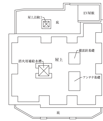
R階平面図
