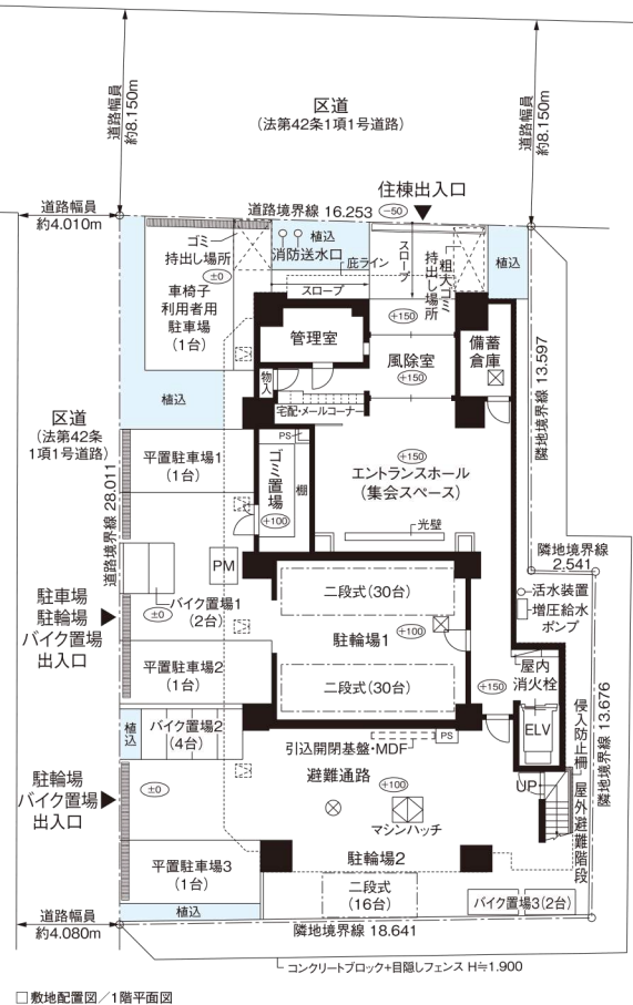
敷地配置図 / 1階平面図
